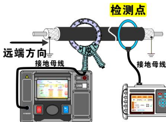
图 6.2 耦合法识别示意图
