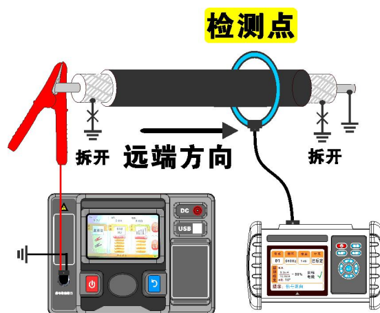
图 5.3 停电电缆识别示意图
